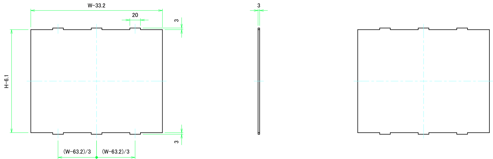
Wパネル1表面 / W Panel 1 Frontside
