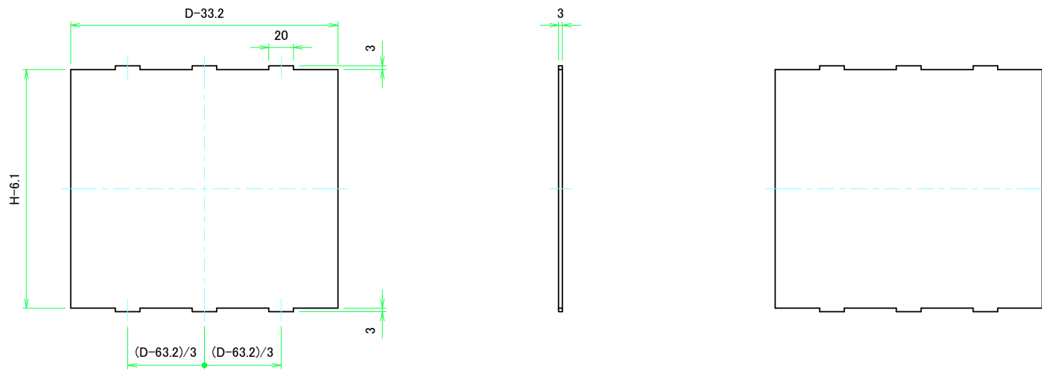
Dパネル1表面 / D Panel 1 Frontside
